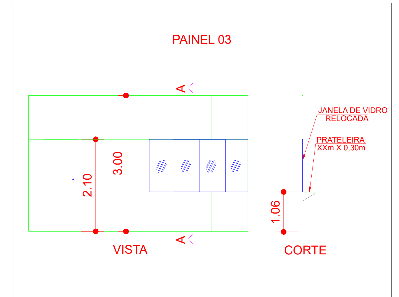
DET 02 ESC:1/100
