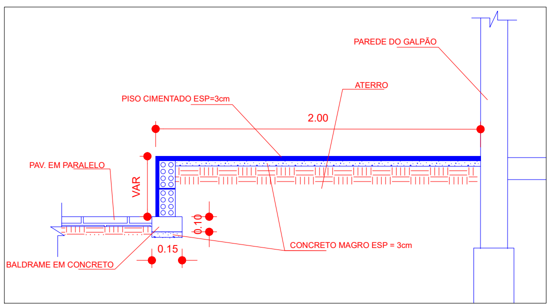
DET. CALÇADA ESC:1/25
