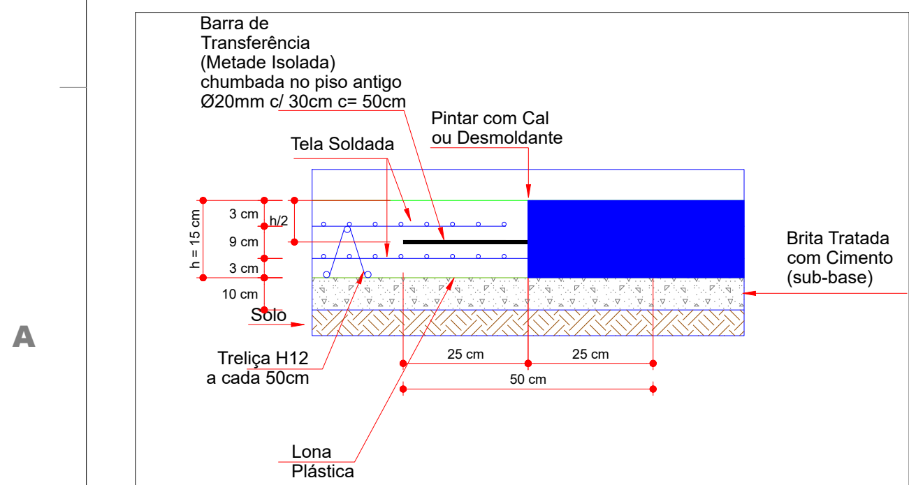
DET. COMPLEMENTO DE PISO ESC:1/20
