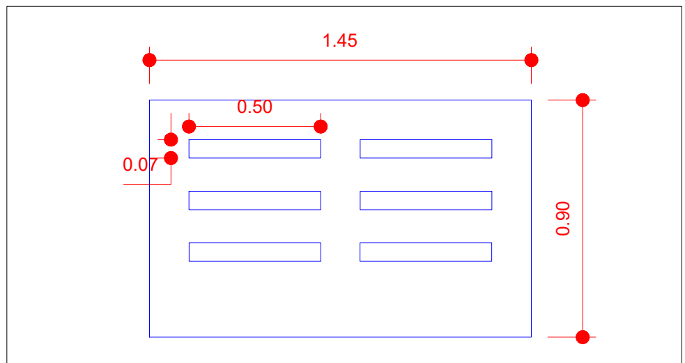
DET. TAMPA DRENAGEM ESC:1/20
