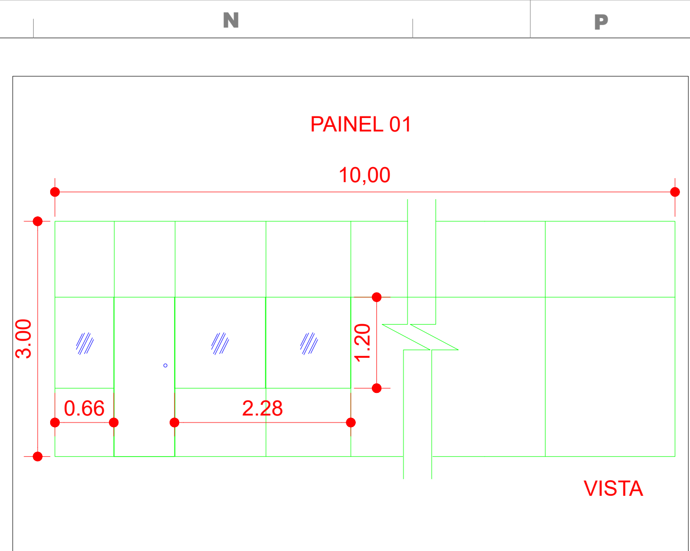
DET 01 ESC:1/100
